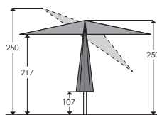
Abmessungen (cm) für Größe 240 x 140 cm:
