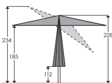
Abmessungen (cm) für Größe 220 cm Ø:
