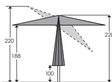
Abmessungen (cm) für Größe 210 x 130 cm:
