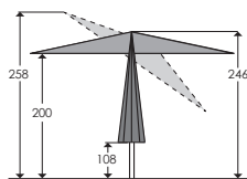
Abmessungen (cm) für Größe 270 cm Ø:
