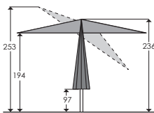
Abmessungen (cm) für Größe 270 cm Ø:
