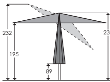
Abmessungen (cm) für Größe 230 x 150 cm:
