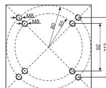
Lochkreis: Angaben in mm
